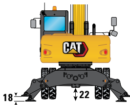
Espacio libre máximo del neumático con el estabilizador completamente abajo
