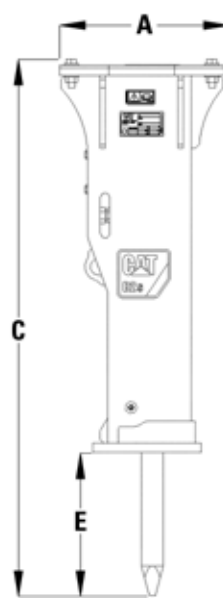
Se muestra el Martillo B2s (silenciado)
