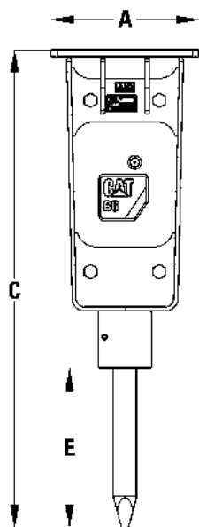
Se muestra el Martillo B6 (no silenciado)
